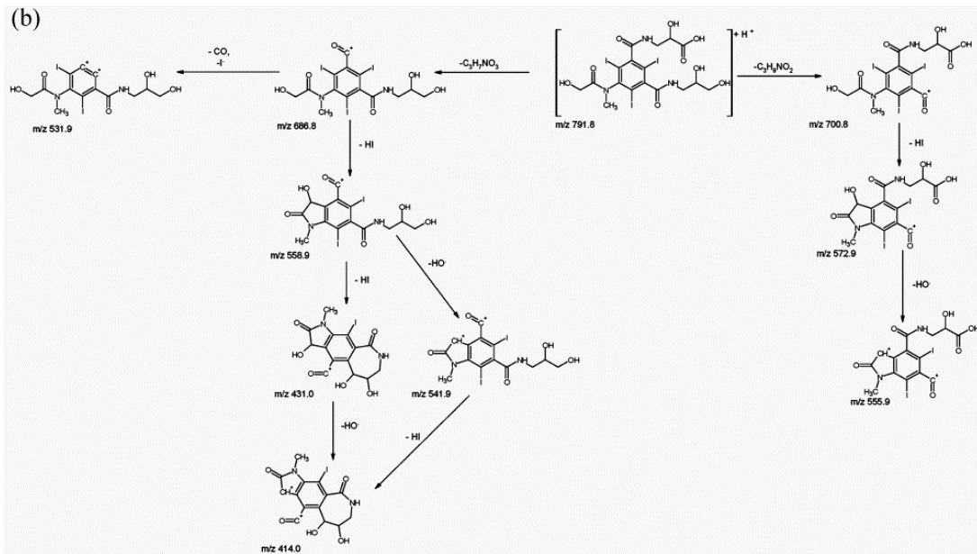
Abb.1 aus Kormos et al. 2010: Vorgeschlagener mikrobieller Transformationsprozess von lomeprol.
